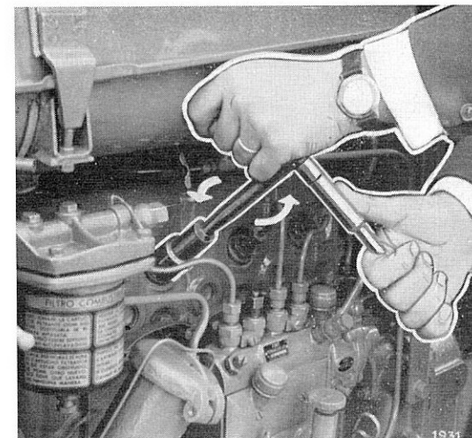
FIG. 21. — Dépose des injecteurs.
