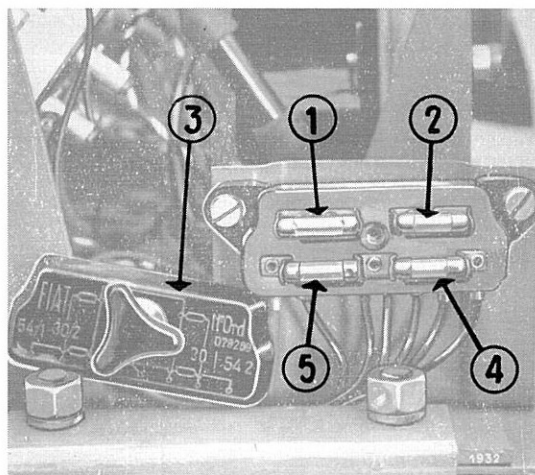
FIG. 23. — Fusibles de protection des appareils d'éclairage.
