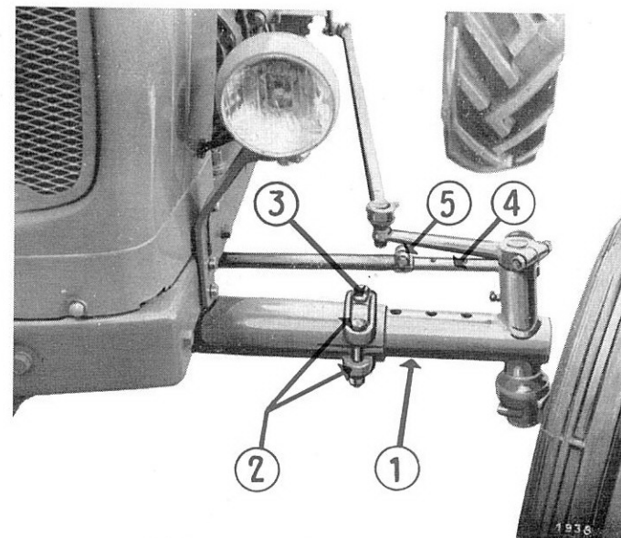
FIG. 9. — Variation de la voie avant
