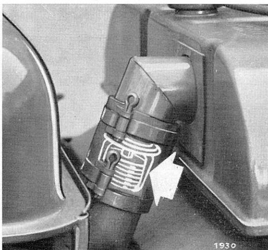
FIG. 19. — Emplacement du thermostat.
