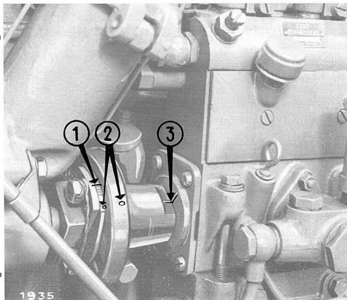
FIG. 28. — Repères sur la pompe d'injection et sur son entraînement.
