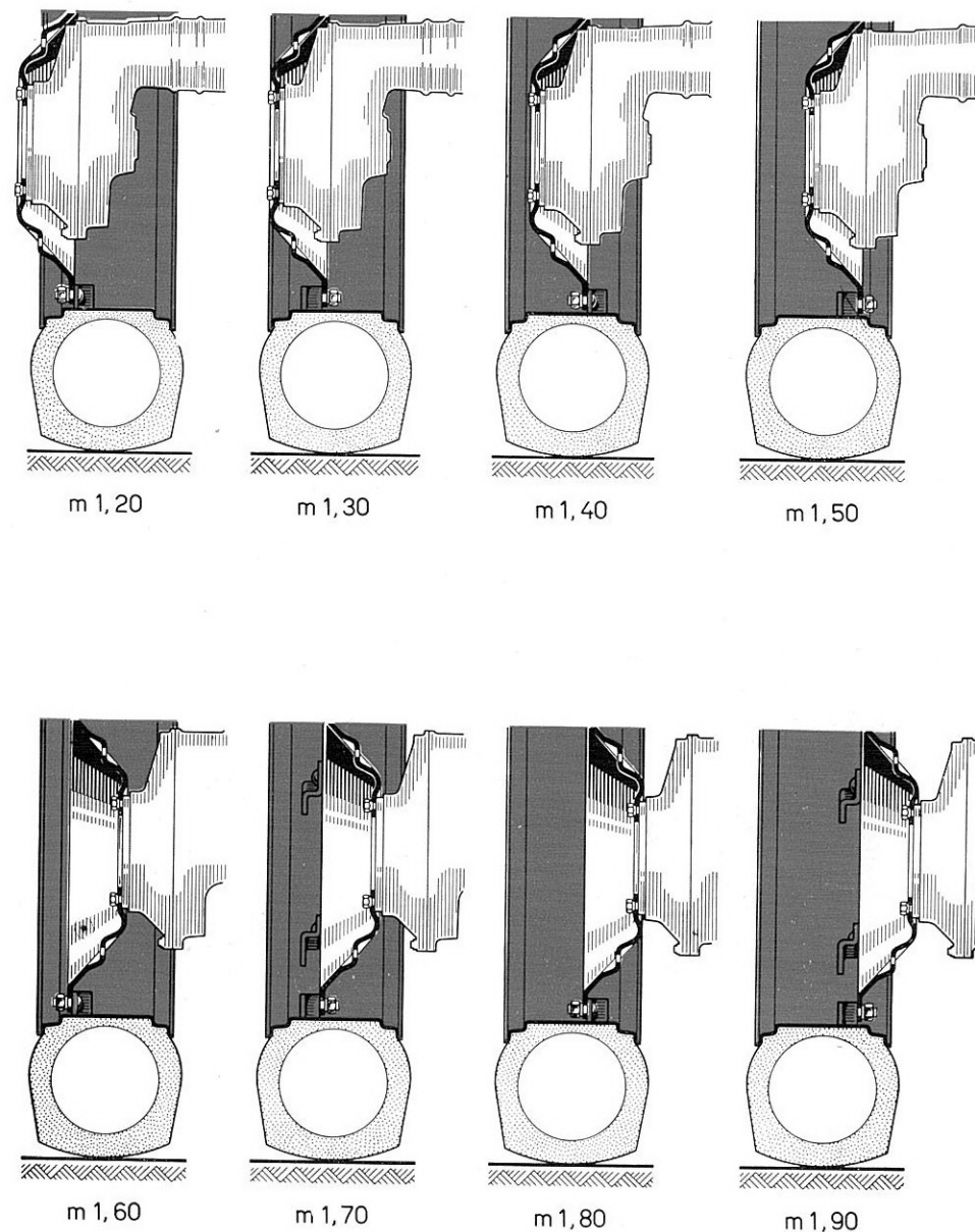
FIG. 10. — Variation de la voie arrière.
