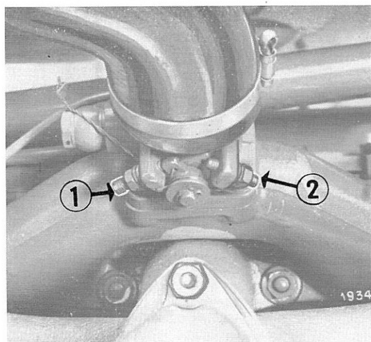
FIG. 25. — Vis de réglage du régime du moteur.
