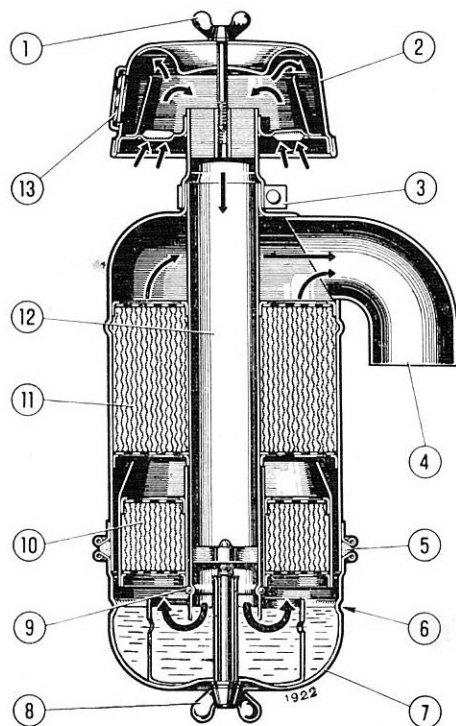
FIG. 17. — Coupe du filtre à air.
