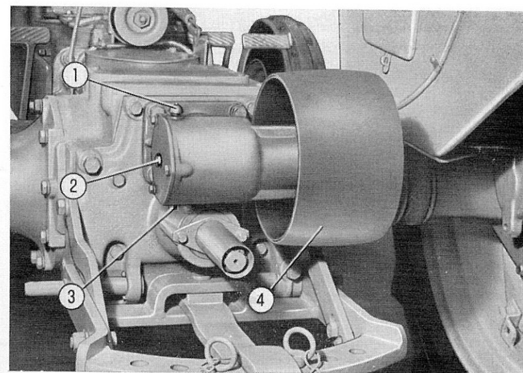
FIG. 32. — Poulie de battage.
