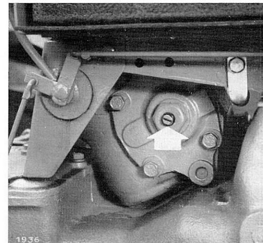
FIG. 30. — Vis de réglage de la commande de direction.
