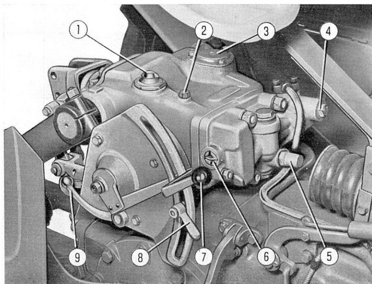
FIG. 11. — Dispositif de relevage
