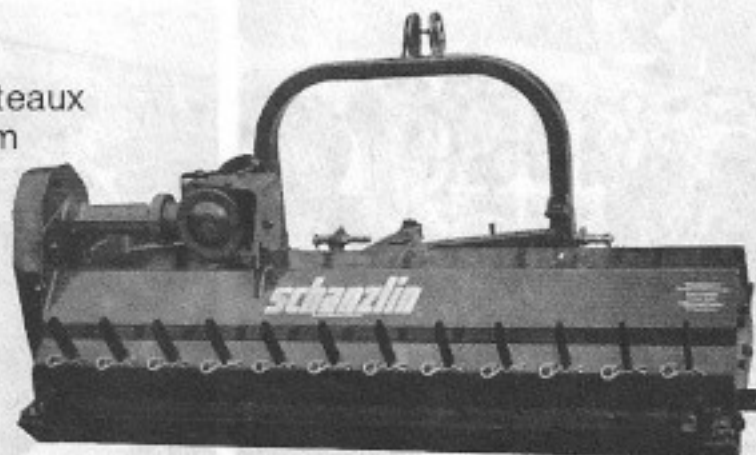
Rogneuse Simple ou Double barre
