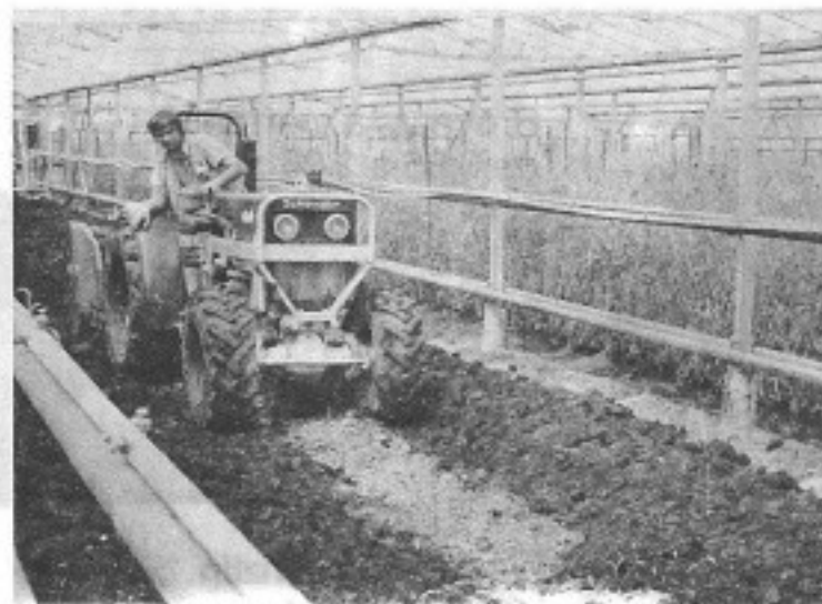
Tracteur avec bêche rotative
