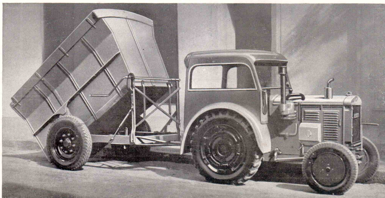
Tracteur 8 CV. "85" Type AFV avec Benne à ordures ménagères
