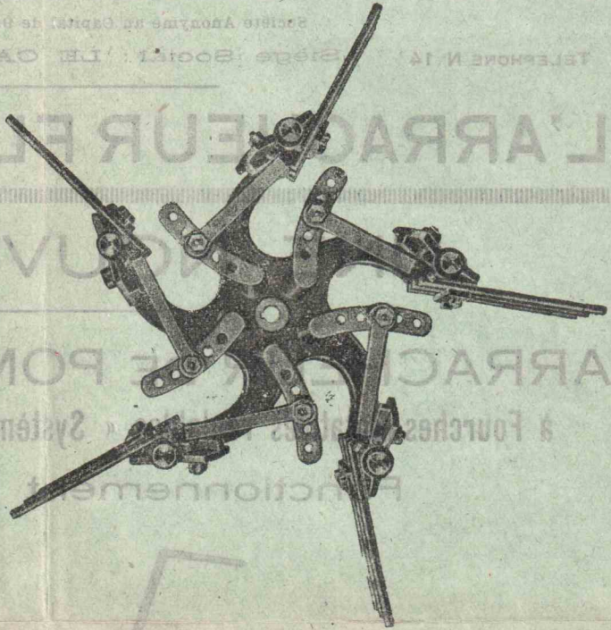
Vue du disque arracheur Système « Vieille »
