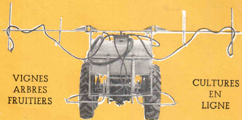
Rampe à vignes 6 SLF 640
