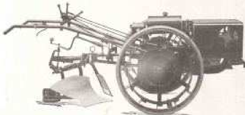
Type C7-7 cv Moteur 4 temps Marche arrière 3 vitesses Prix ..... 8.500 fr.
