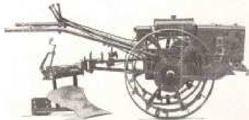
Type B6-5 cv. Moteur 2 temps, marche arrière Prix ..... 6.850 fr.
