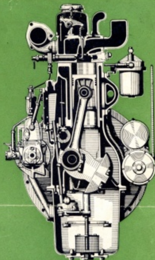
Coupe du moteur diesel PANHARD, type 4 H L équipant le CP 60 N
