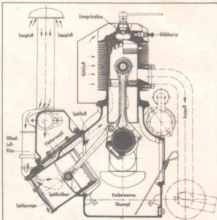
Querschnitt durch den luftgekühlten Motor des NORMAG-KORNETT II.
