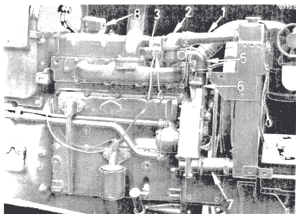
Fig. 44 - Eléments du système de refroidissement 1. Durite d'entrée d'eau dans le radiateur - 2. Thermostat - 3. Collecteur d'eau - 4. Prise de température - 5. By-pass - 6. Pompe à eau - 7. Durite de sortie d'eau de radiateur - 8. Régulateur de tension -
