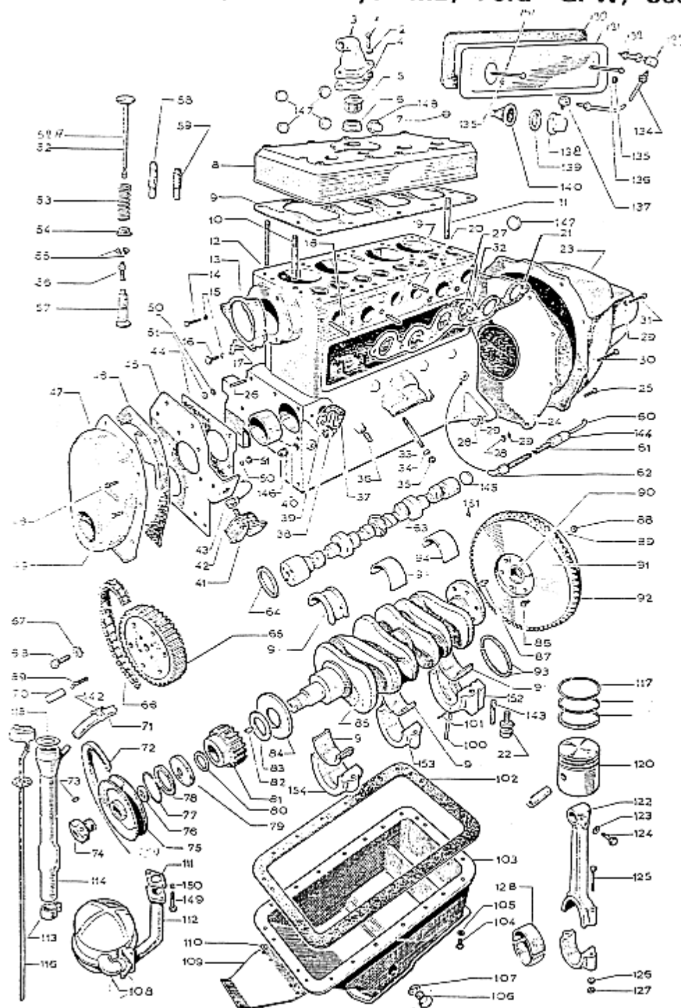
Motor
