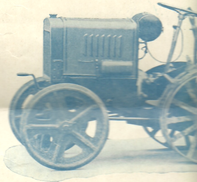
Tracteur DAVID équipé avec son brabant Roues sans bandages caoutchouc. Les crampons, toutefois, sur demande et pour les terrains.
