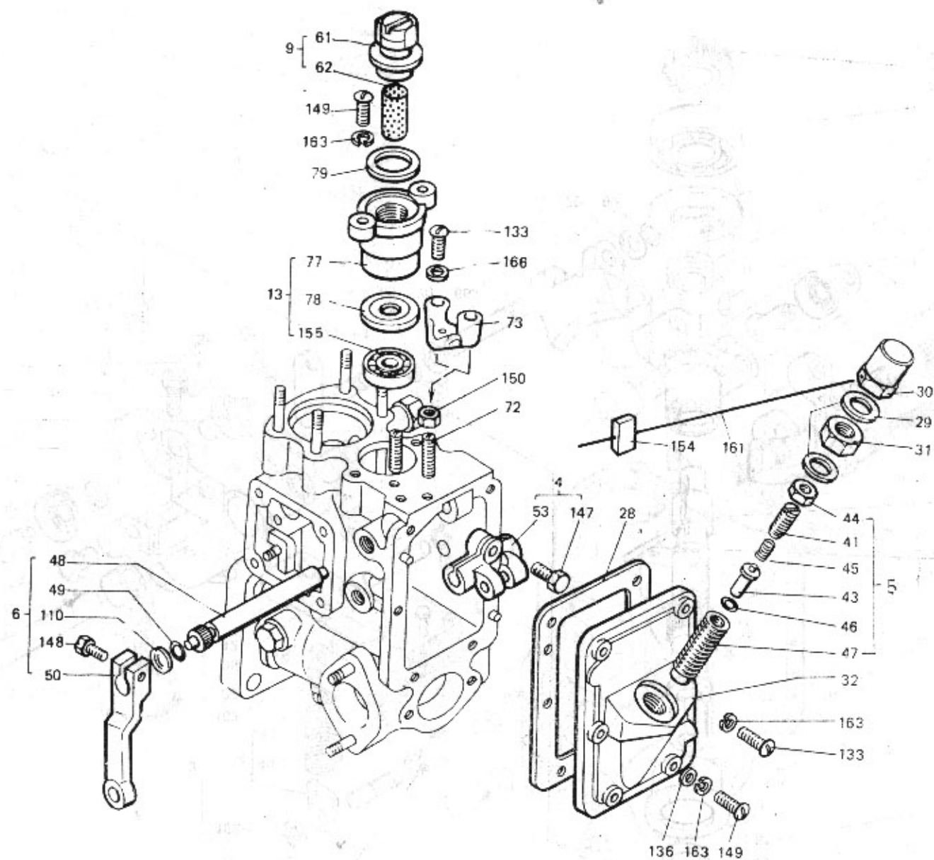
Р и с. 33. Насос топливный распределительный односекционный 54.1111004-50
