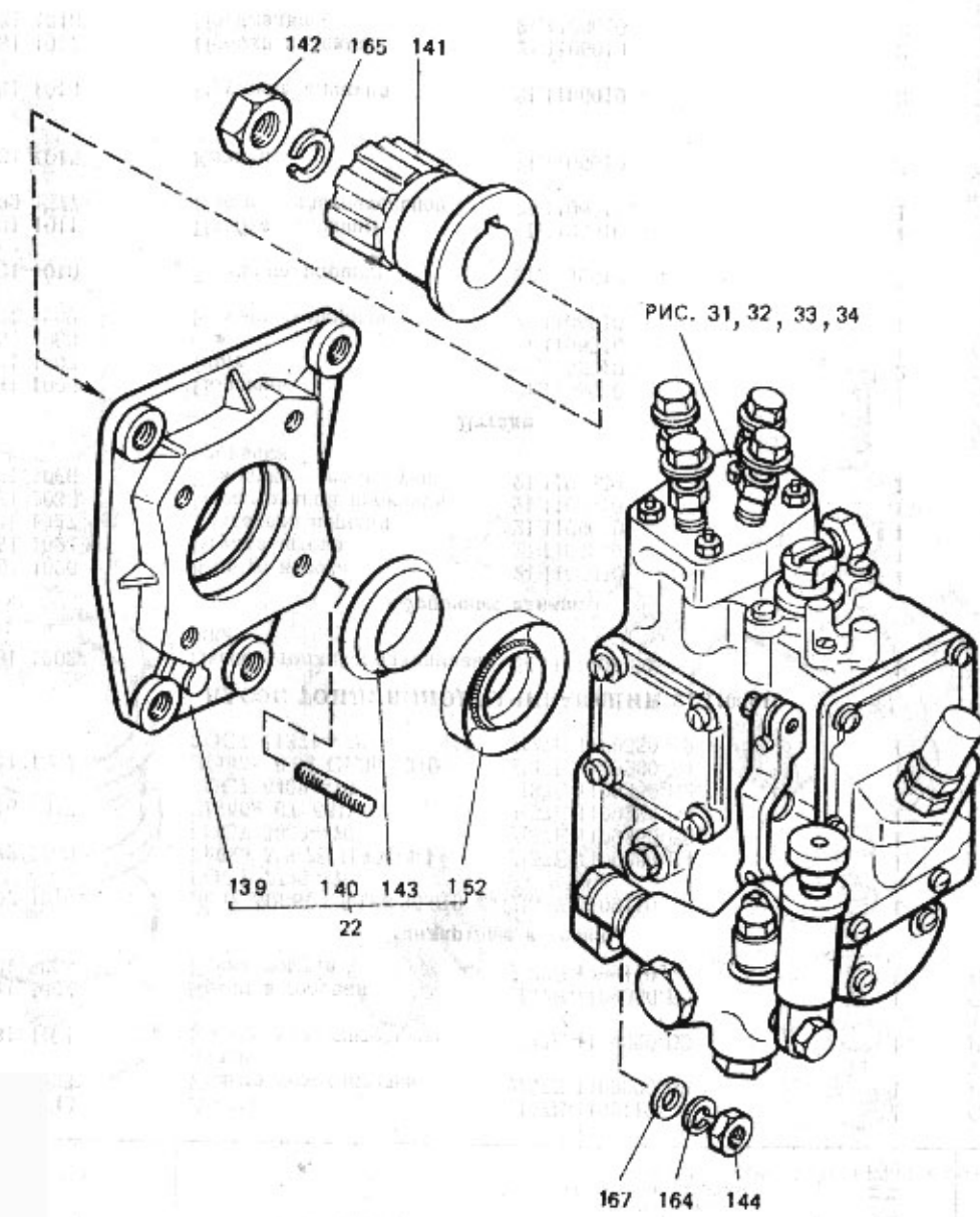
Рис. 30. Насос топливный распределительный односекционный 54.1111004-50
