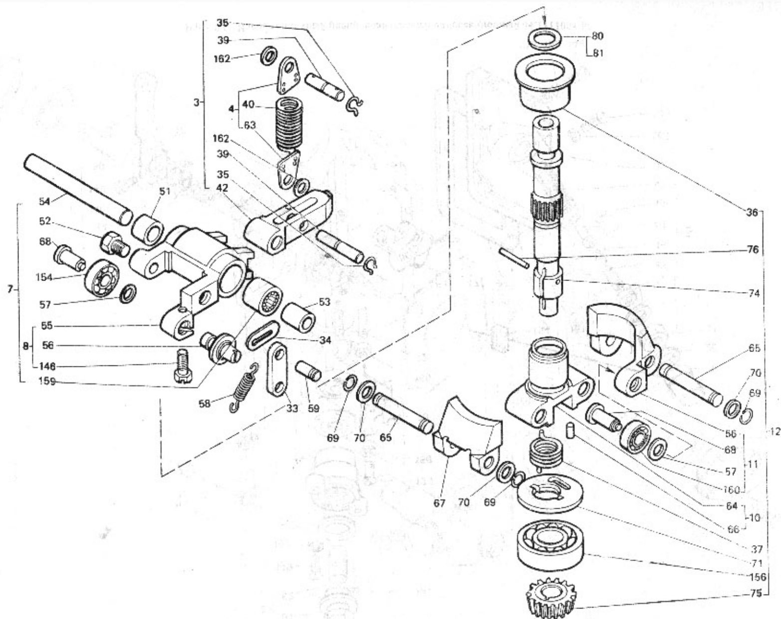
Рис. 32. Насос топливный распределительный односекционный 54.1111004-50
