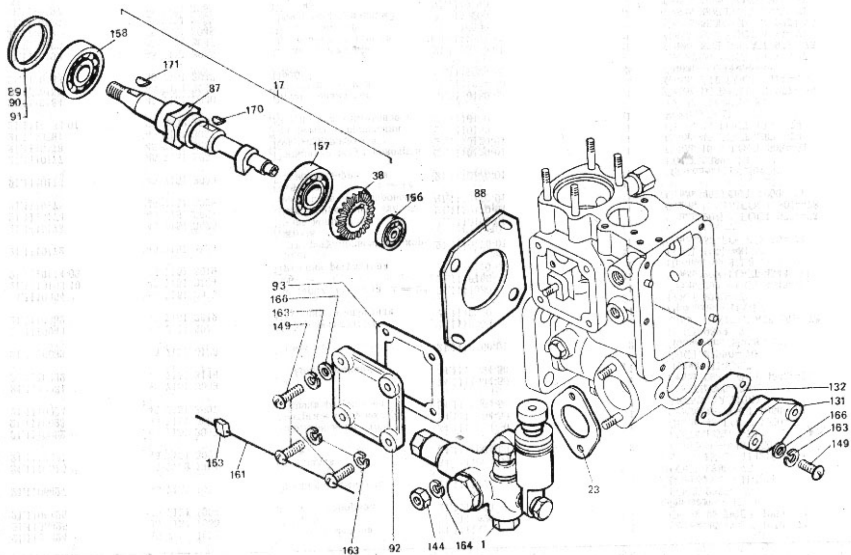
Р и с. 34. Насос топливный распределительный односекционный 54.1111004-50
